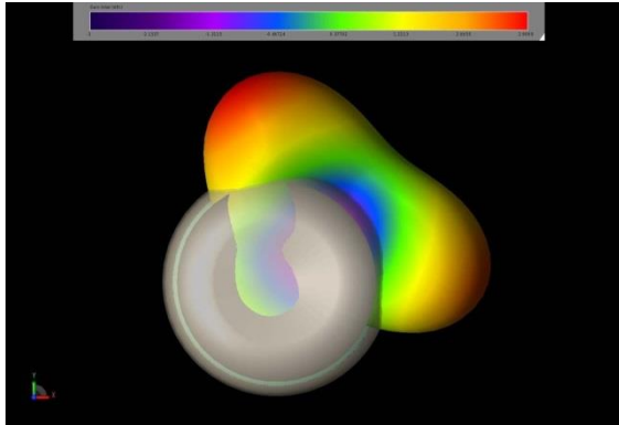
図6：2.4 GHzアンテナ1基の放射パターン上面図 水平面に集束した2つのローブがある。
