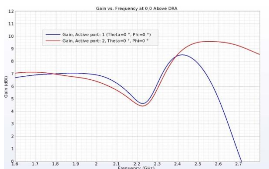
図5：デュアルバンドアンテナの直上の点における利得
