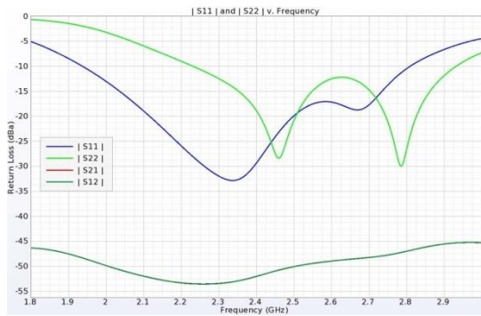
図17：広帯域アンテナのSパラメータ どちらのポートからの給電においても、2.25～2.8GHzの範囲でリターンロスが-10dB以下となり、対象となる帯域以上をカバーしている 2ポート間のアイソレーションは-45dB以下となっている
