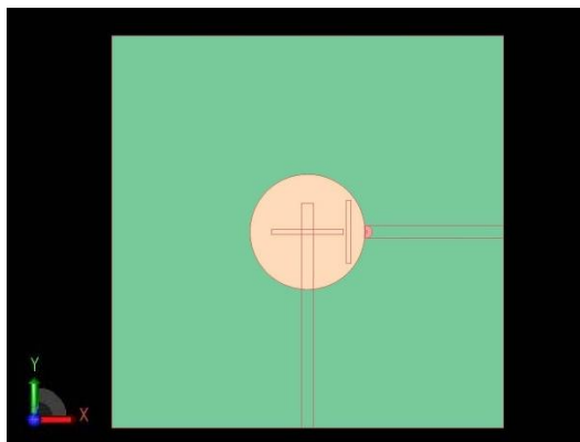
図2：デュアルバンドアンテナの上面図 2本のMSLと、2つのスロットと同軸プローブが示されている
