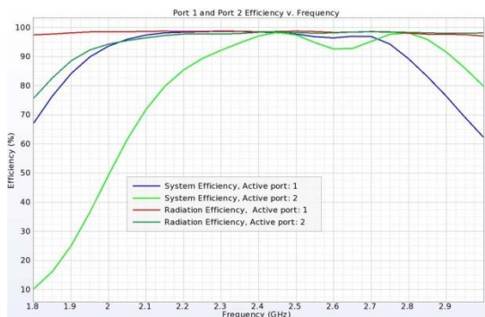
図19：広帯域アンテナの放射効率とシステム効率 この広帯域アンテナは非常に効率的で、対象となる帯域でミスマッチ損失含むシステム効率が100%近くになっている
