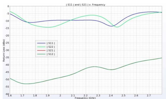
図4：デュアルバンドアンテナのSパラメータ 1.71~1.88GHzと2.4~2.48GHzの範囲で動作する領域を示している ポート間のアイソレーションは35dB以下
