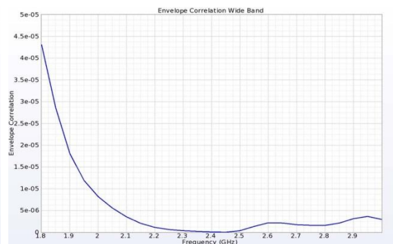
図20：広帯域アンテナのエンベロープ相関値 エンベロープ相関は極めて低く、2つのポートの利得パターン間のアイソレーションが非常に良好であることを示している
