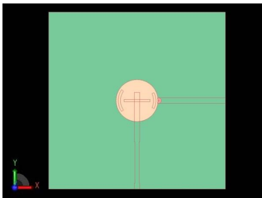
図3：広帯域アンテナの上面図
